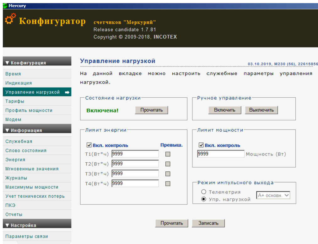
Рисунок 5.12 – Вкладка «Управление нагрузкой»
