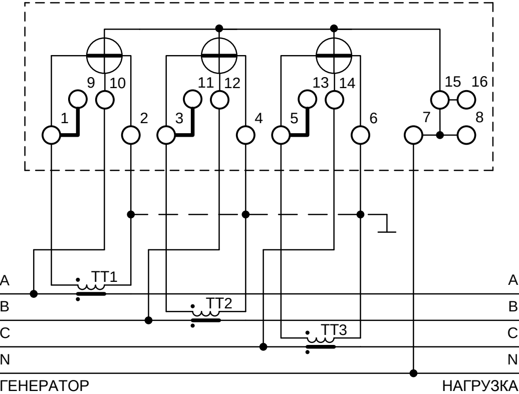
Рисунок Б.2 – Схема подключения через три трансформатора тока
