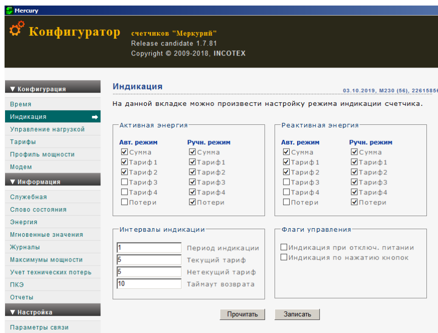
Рисунок 5.4 – Вкладка «Индикация»
