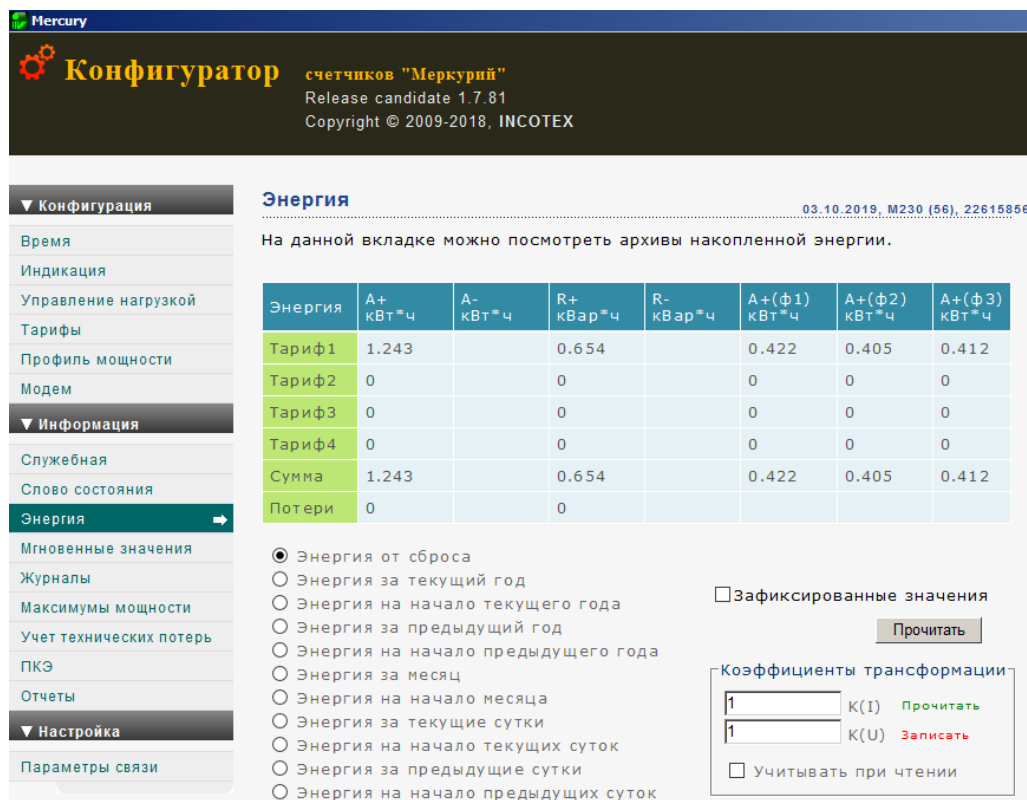
Рисунок 5.7 – Вкладка «Энергия»
